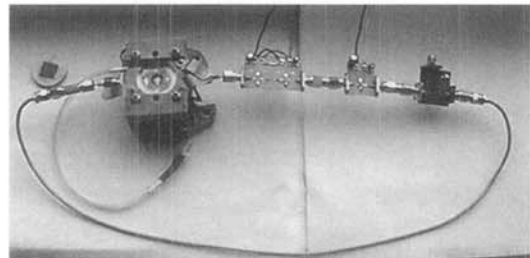
그림 7. 제작된 발진기. Fig. 7. The fabricated oscillator.
