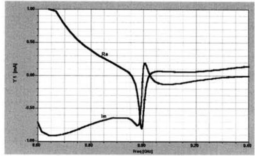
(a) 발진기의 부성저항 특성 (a) The negative resistance characteristic
