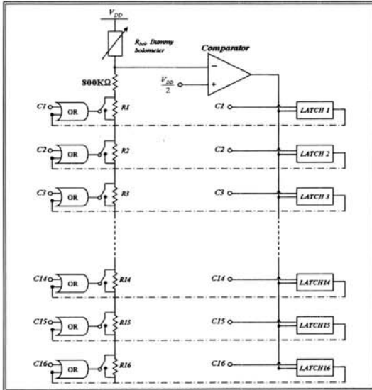
그림 1. 기준저항 보상회로.
