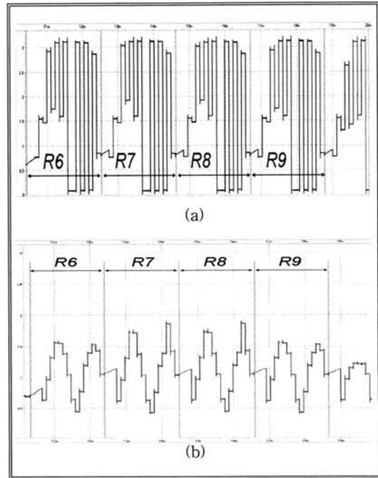
그림 3. 출력파형 비교 (a)기존 검출 회로, (b)제안한 검출회로.
