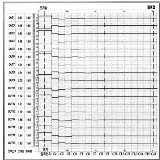
그림 4. 보상 입력신호 시뮬레이션 결과.
