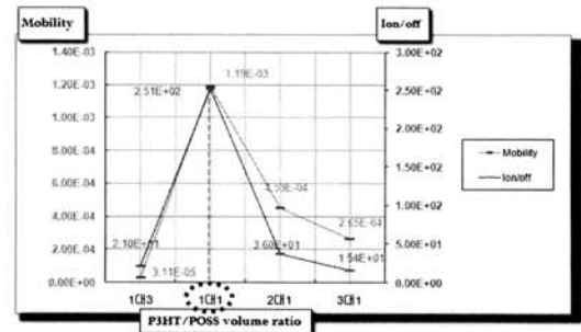
그림 6. P3HT와 POSS의 부피비에 따른 이동도와 전류점멸비의 변화. Fig. 6. Mobility and I_{on/off} ratio variations with different P3HT/POSS volume ratios.
