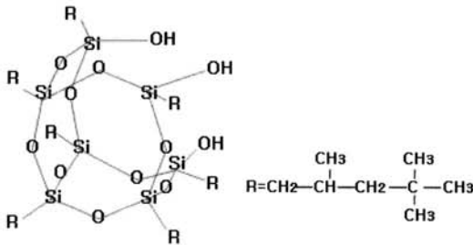
그림 2. POSS의 화학적 구조. Fig. 2. Chemical structure of POSS.
