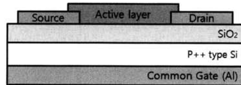
그림 3. 제작된 하부전극구조를 갖는 OTFT의 단면구조. Fig. 3. Schematic diagram of an OTFT with Bottom Contact (BC) configuration.
