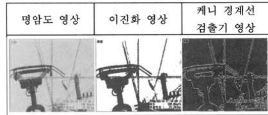
그림 5. 이진화 처리를 통한 전처리 과정. Fig. 5. Pre-processing with binary image.
