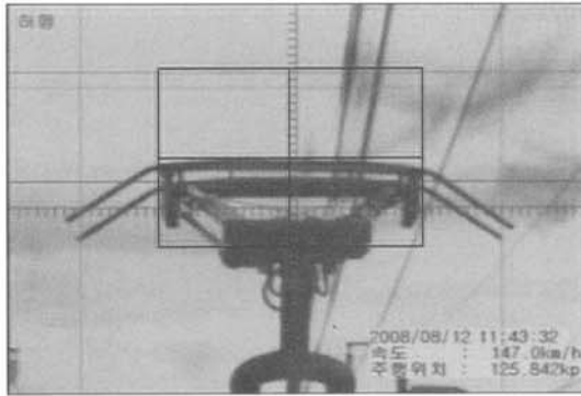
그림 2. 팬터그래프-전차선 동편위 측정 영상. Fig. 2. Image of pantograph-catenary dynamic stagger measurement.
