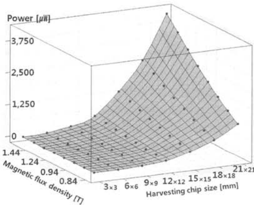
그림 5. 칩크기와 자속밀도에 따른 발생전력.
