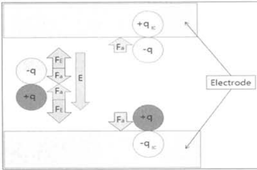
그림 2. 셀 내부에 작용하는 힘. Fig. 2. Attractive force in a cell.
