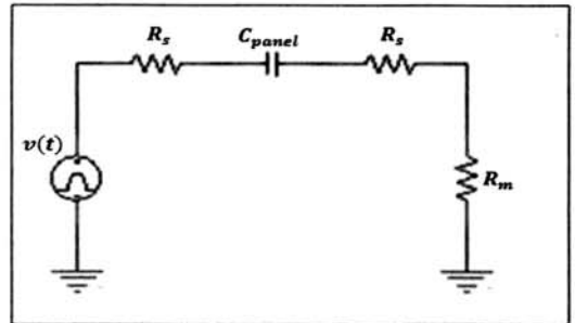
그림 6. 전류측정을 위해 구성된 등가회로. Fig. 6. Equivalent circuit of current detection.
