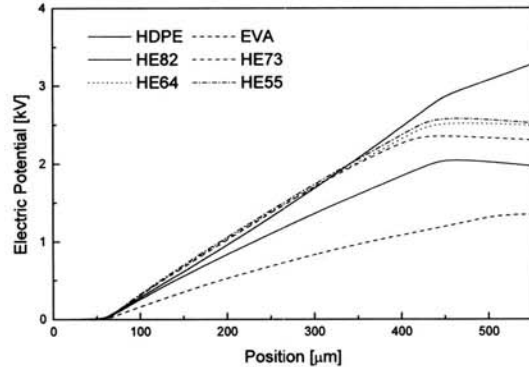
(b) 전위분포
