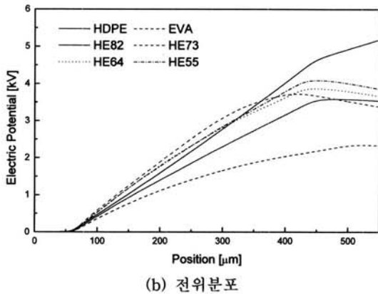
그림 4. 각시편의 전계 및 전위분포(DC 5 kV인가). Fig. 4. Electric field and potential distribution in specimens at DC 5 kV.
