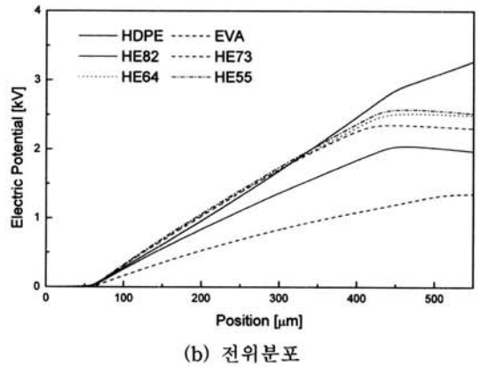
그림 5. 10분후의 전계 및 전위분포(DC 3 kV인가). Fig. 5. Electric field and potential distribution in specimens after 10 minutes at DC 3 kV.
