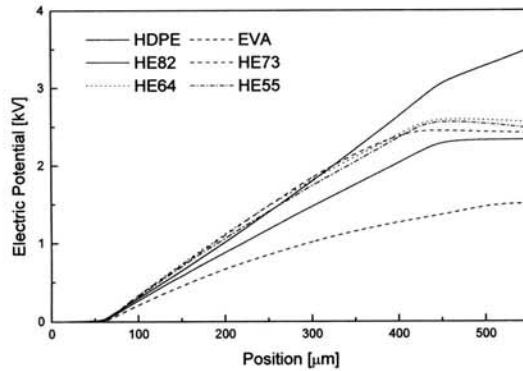
(b) 전위분포
