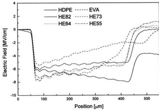
(a) 전계분포
