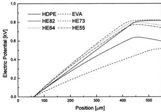
(b) 전위분포
