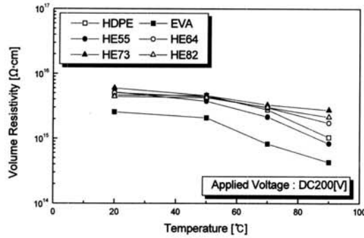
그림 9. 체적저항율의 온도의존성(DC 200 V일 때). Fig. 9. Temperature dependency of volume resistivity(Applied Voltage : DC 200 V).
