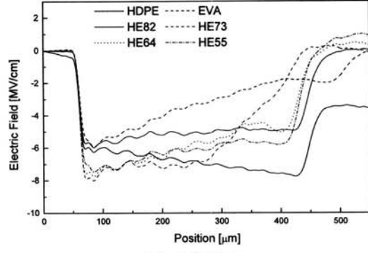
(a) 전계분포
