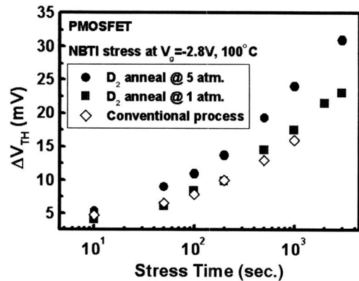
그림 3. 중수소 열처리된 PMOSFET의 NBTI 스트레스에 대한 문턱 전압의 변화.
