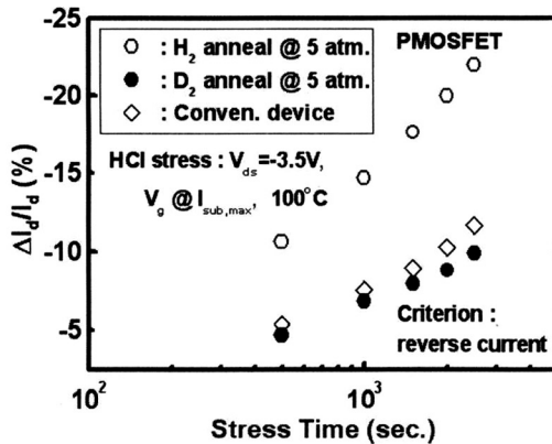
그림 8. 수소 및 중수소 열처리된 PMOSFET의 HCl 스트레스에 대한 포화 전류의 감소. Fig. 8. Decrease of saturation current depending on HCl stress time for both hydrogen and deuterium annealed PMOSFETs.
