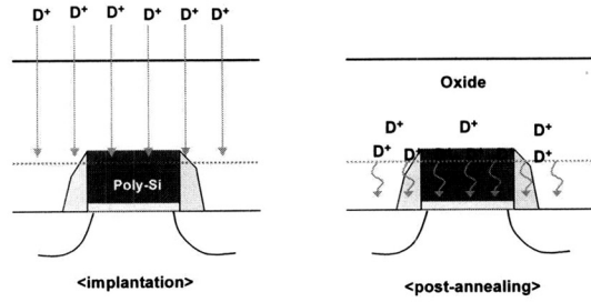
그림 11. 제안된 저에너지 중수소 이온 주입법의 개략도.
