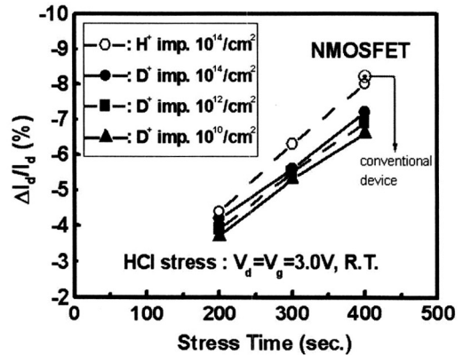
그림 9. 수소 및 중수소 이온 주입된 NMOSFET의 HCl 스트레스에 대한 포화 전류의 감소. Fig. 9. Decrease of saturation current depending on HCl stress time for both hydrogen and deuterium implanted NMOSFETs.
