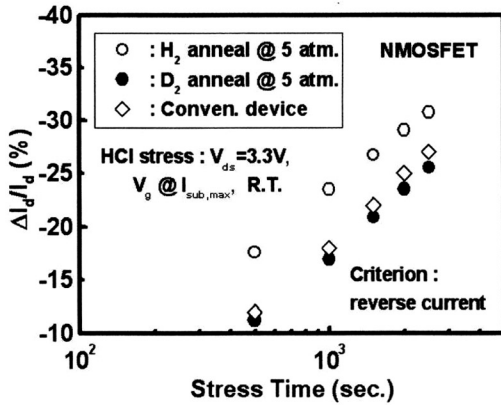
그림 7. 수소 및 중수소 열처리된 NMOSFET의 HCl 스트레스에 대한 포화 전류의 감소. Fig. 7. Decrease of saturation current depending on HCl stress time for both hydrogen and deuterium annealed NMOSFETs.
