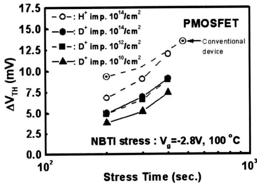
그림 5. 중수소 이온 주입된 PMOSFET의 NBTI 스트레스에 대한 문턱 전압의 변화.
