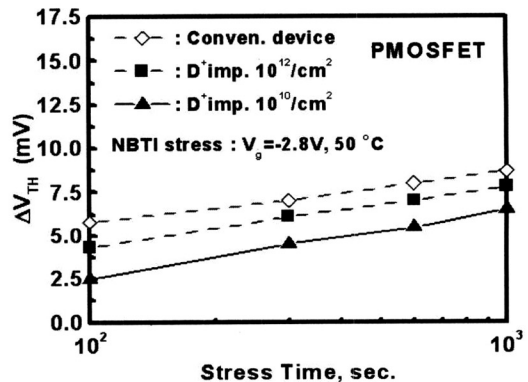
그림 6. 중수소 이온 주입된 PMOSFET의 NBTI 스트레스 ( 50^\circ\text{C} )에 대한 문턱 전압의 변화.
