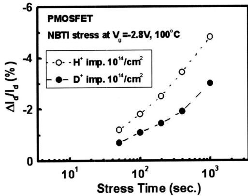
그림 4. 수소 및 중수소 이온 주입된 PMOSFET의 NBTI 스트레스에 대한 포화 전류의 감소.
