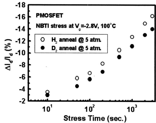
그림 2. 수소 및 중수소 열처리된 PMOSFET의 NBTI 스트레스에 대한 포화 전류의 감소.
