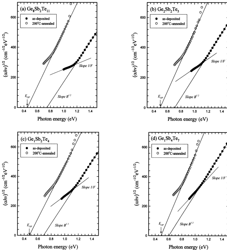
그림 5. 증착직후(●) 및 200 °C 열처리(○) (GeTe) x (Sb 2 Te 3 )박막에 대한 h\nu vs (\alpha h\nu)^{1/2} 그래프 : (a) Ge 8 Sb 2 Te 11 , (b) Ge 2 Sb 2 Te 5 , (c) Ge 1 Sb 2 Te 4 , (d) Ge 1 Sb 4 Te 7 .
