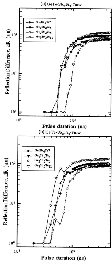
그림 9. (a) 7 mW 및 (b) 9 mW 에서 측정된 (\text{GeTe})_x(\text{Sb}_2\text{Te}_3) 박막의 결정화 형성에 따른 반사도 변화.
