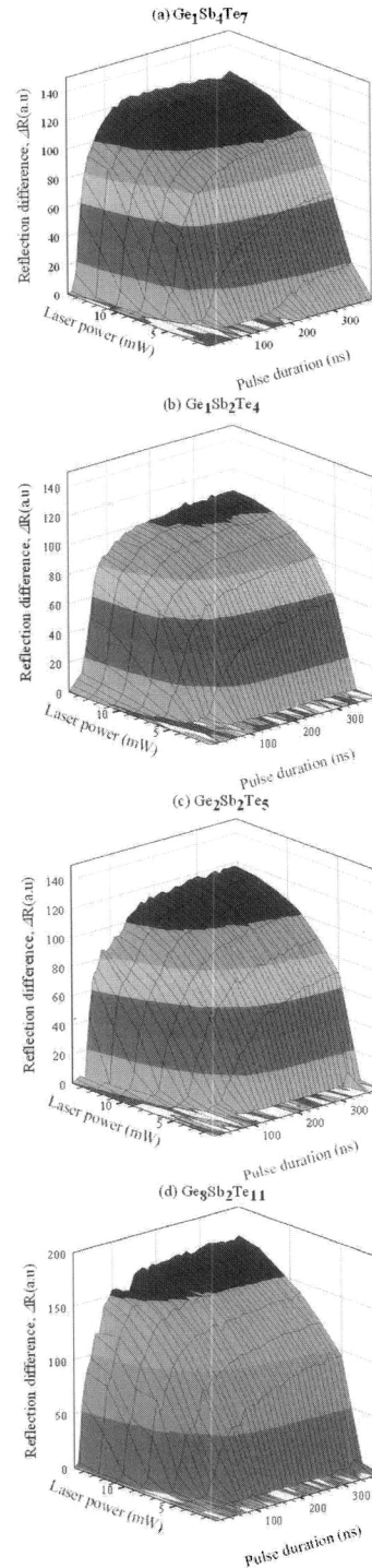
그림 7. (GeTe) x (Sb 2 Te 3 )의 결정화 형성에 따른 반사도 변화에 대한 3D-mesh plot.
