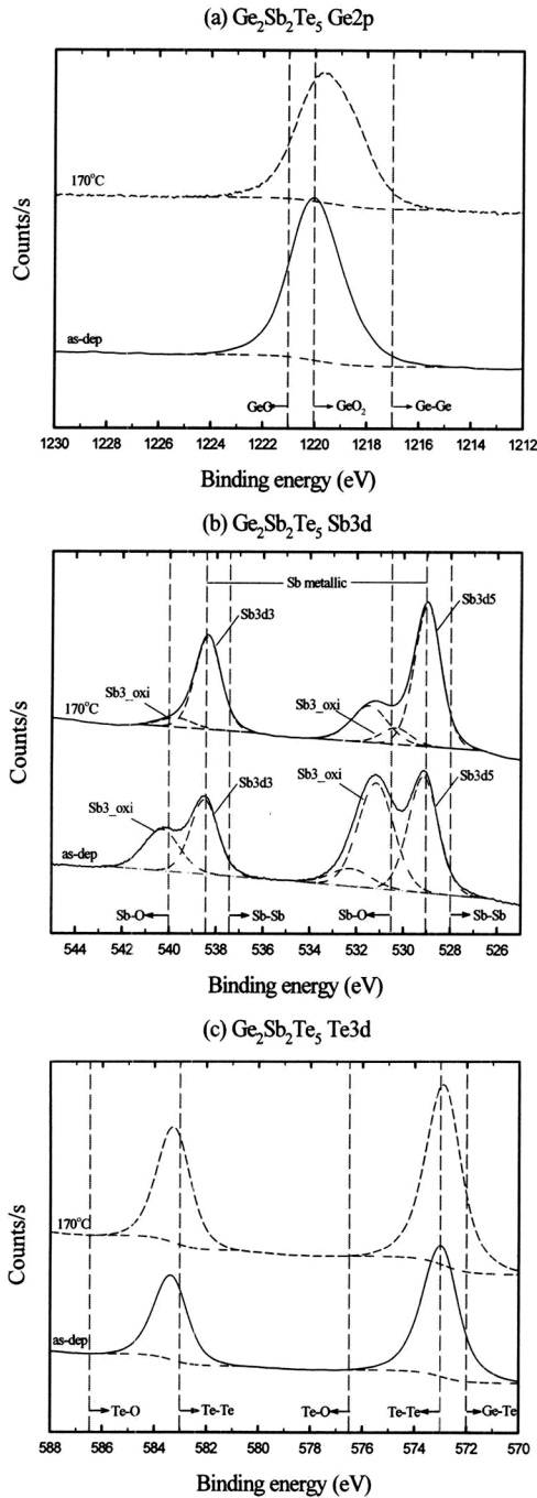
그림 3. 증착직후 및 170 °C 열처리 \text{Ge}_2\text{Sb}_2\text{Te}_5 박막의 XPS 스펙트라 : (a) Ge2p, (b) Sb3d, (c) Te3d.
