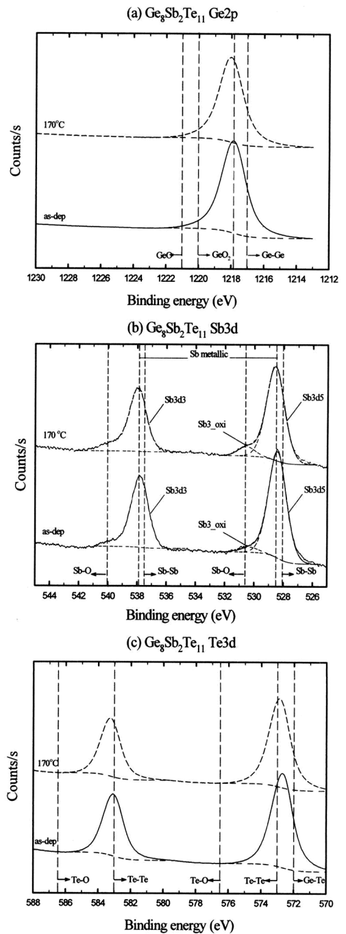
그림 4. 증착직후 및 170 °C 열처리 \text{Ge}_8\text{Sb}_2\text{Te}_{11} 박막의 XPS 스펙트라 : (a) Ge2p, (b) Sb3d, (c) Te3d.
