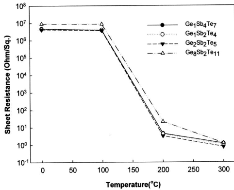
그림 6. (GeTe) x (Sb 2 Te 3 ) 박막의 열처리 온도에 따른 면저항 변화.
