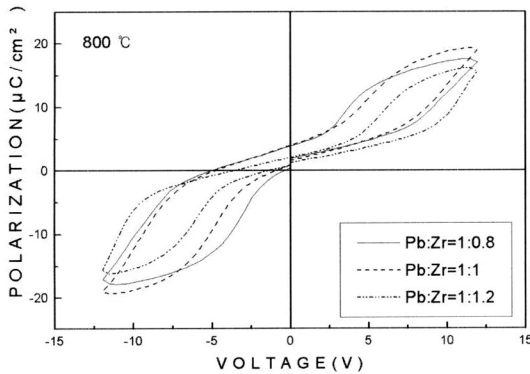
그림 4. 800 °C에서 몰 비에 따른 이력곡선. Fig. 4. Hysteresis curve with different mole ratio of PbZrO 3 films annealed at 800 °C.
