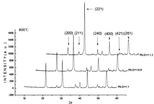
그림 1. 800 °C의 Pb와 Zr의 몰 비에 따른 XRD. Fig. 1. XRD with different mole ratio of PbZrO 3 films annealed at 800 °C.
