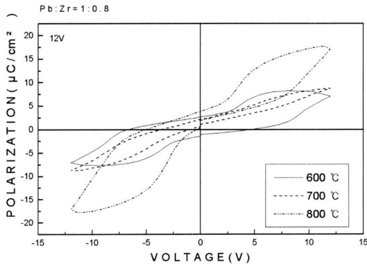
그림 3. Pb:Zr=1:0.8에서 온도에 따른 이력곡선. Fig. 3. Hysteresis curve with different annealing temperature of PbZrO 3 films that mole ratio of Pb:Zr.
