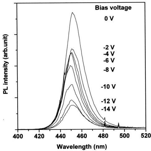
그림 2. 바이어스 전압의 변화에 따른 PL 스펙트럼. 역방향 전압이 커지며 크기는 작아지고, peak 위치는 blue-shift 후 red-shift 함을 보여준다.
