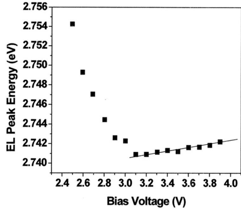
그림 4. 바이어스 전압의 변화에 따른 EL peak 에너지의 변화. 순방향 전압이 커지며 QCSE 때문에 에너지가 감소하다가 band bending이 끝나는 built-in 전압과 같은 위치에서 에너지 변화가 적어진다.
