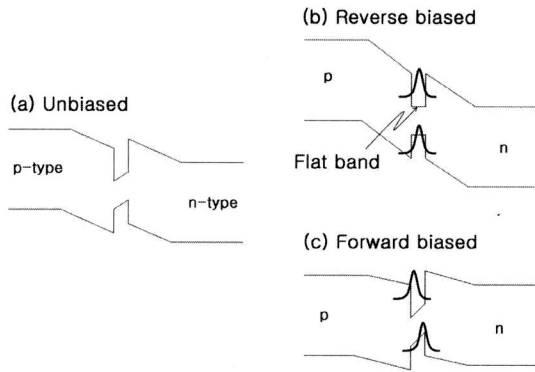
그림 1. pn 다이오드 구조의 바이어스 전압에 따른 에너지 밴드 그림. (a) 전압이 걸리지 않았을 때, (b) 알맞은 역방향 전압이 걸려 flat band가 되었을 때, (c) 순방향 전압이 걸렸을 때. 양자 우물 내의 곡선은 전자와 정공의 파동 함수를 나타낸다.
