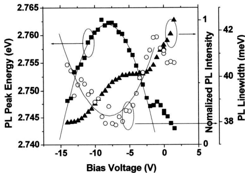
그림 3. 바이어스 전압에 따른 PL peak 에너지 (네모), PL 크기 (세모), PL peak의 폭 (원)의 변화. 실선들은 이차함수로 근사된 결과이다.
