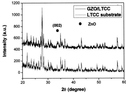
그림 3. 제작한 박막의 X선 회절 패턴. Fig. 3. X-ray diffraction pattern of the fabricated thin film.
