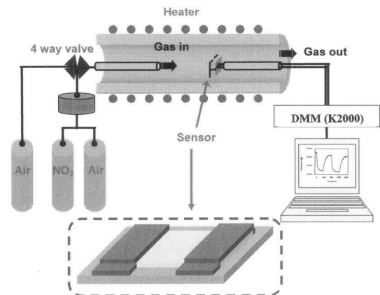
그림 2. NO x 가스 측정시스템. Fig. 2. Measurement system for NO x gas.
