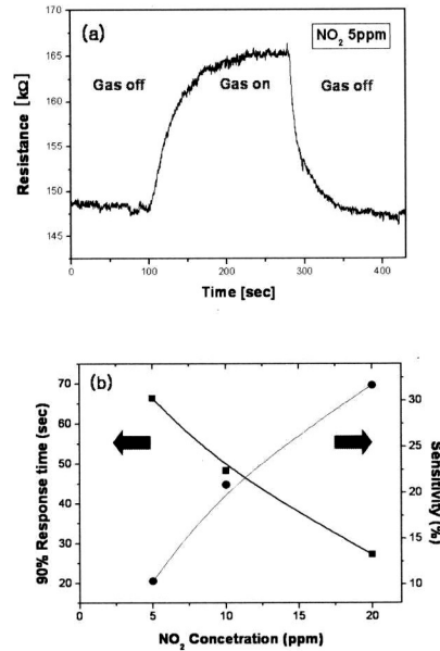
그림 5. 가스농도에 따른 센싱 특성에 대한 측정 결과. Fig. 5. Sensing characteristics under different NO 2 concentration.
