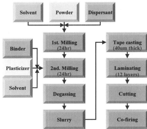
그림 1. LTCC 기판 제조공정. Fig. 1. Fabrication process for LTCC substrate.
