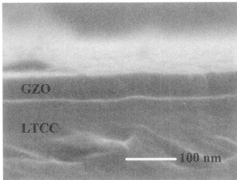
그림 4. 제작한 박막의 FESEM 이미지. Fig. 4. FESEM image of the fabricated thin film.
