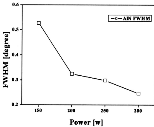
그림 2. 전력에 따른 AlN 박막의 FWHM 값. Fig. 2. FWHM pattern of AlN films at different RF power.
