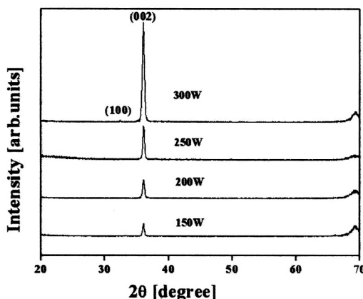
그림 1. 전력에 따른 AlN 박막의 X선 회절 패턴. Fig. 1. XRD pattern of AlN films at different RF power.
