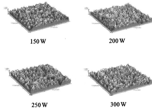
그림 4. AFM 3차원 이미지. Fig. 4. Three-dimensional AFM images of various AlN films.
