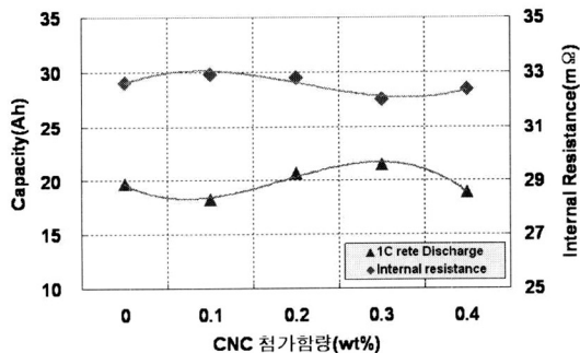
그림 14. CNC함량에 따른 1C을 방전용량 및 내부저항.
