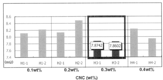
그림 16. CNC 함량에 따른 내부저항.
