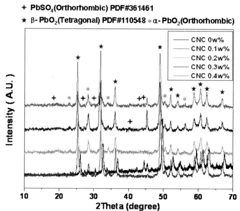
그림 9. CNC함량에 따른 화성극판의 XRD 분석 결과.
