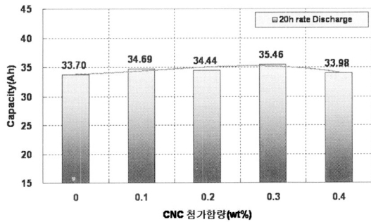
그림 13. CNC함량에 따른 20h을 방전용량.
