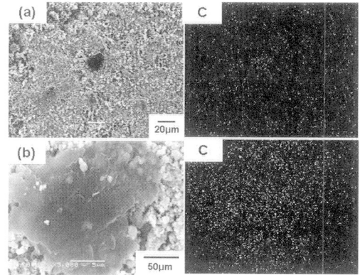
그림 12. CNC가 첨가된 화성극판의 EDS에 의한 Carbon 분포. Fig. 12. EDS mapping image of fotation electrode of CNC additive
