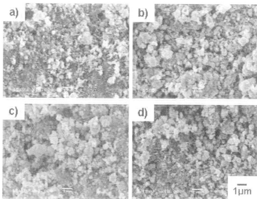
그림 11. CNC함량에 따른 화성극판의 표면형상 관찰. Fig. 11. SEM image of fotation electrode of according to amount CNC in electrode : (a) CNC 0.1 wt%, (b) CNC 0.2 wt%, (c) CNC 0.3 wt%, (d) CNC 0.4 wt%.
