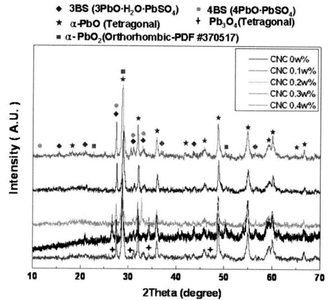
그림 8. CNC함량에 따른 숙성극판의 XRD 분석 결과.
