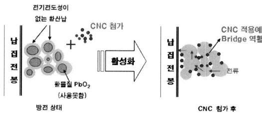
그림 7. 납축전지의 CNC작용원리. Fig. 7. Mechanism for applying CNC to lead acid battery.
