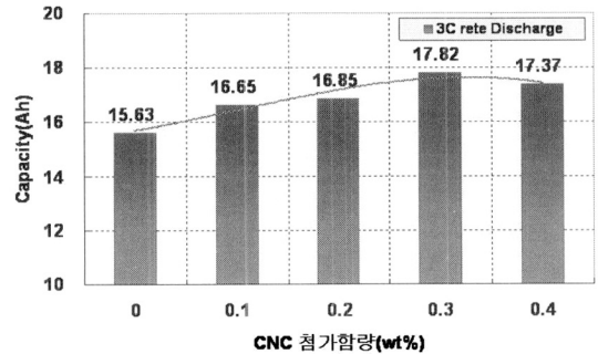
그림 15. CNC함량에 따른 3C을 방전용량 그래프.
