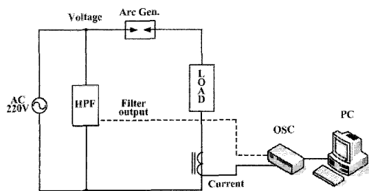
그림 5. 실험계의 구성.
