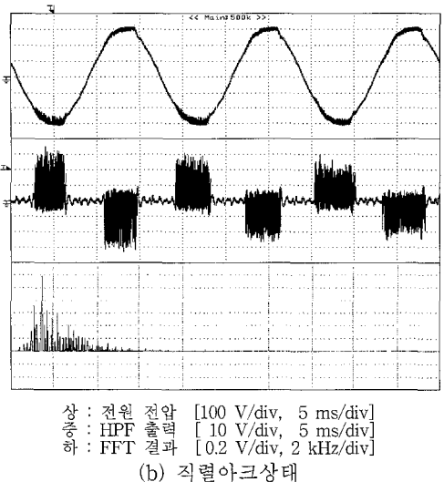
그림 8. 조광부하에서 직렬아크방전. Fig. 8. Series arc discharge in a dimming load.
