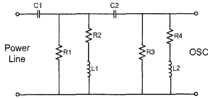
(a) 회로
