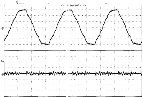
상 : 전원 전압 [ 00 V/div, 5 ms/div] 하 : HPF 출력 [ 10 V/div, 5 ms/div]
