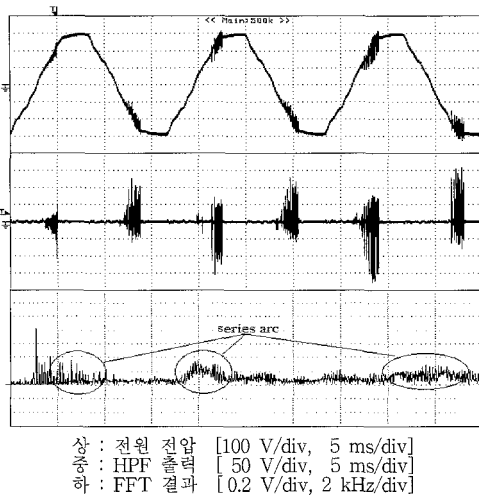
그림 7. 진공청소기에서 직렬아크방전. Fig. 7. Series arc discharge in a vacuum cleaner.
