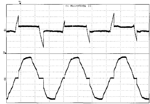
그림 2. 직렬아크 전압 및 전류 파형. Fig. 2. Waveforms of series arc voltage and current.
