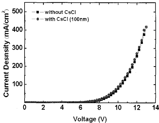
그림 3. Ca/Ag 음극 위에 CsCl 보호막이 증착된 전면발광 OLED의 전류밀도-전압 곡선.
