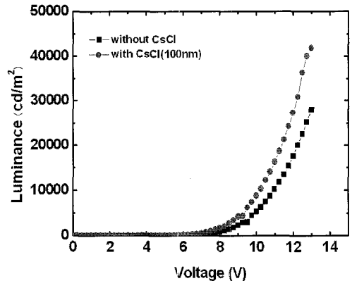
그림 4. Ca/Ag 음극 위에 CsCl 보호막이 증착된 전면발광 OLED의 휘도-전압 곡선.
