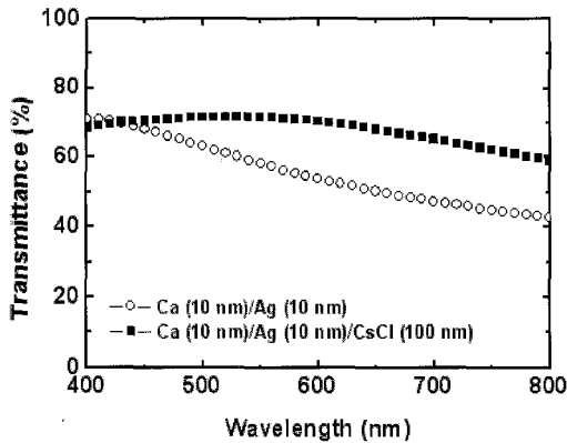
그림 2. Ca/Ag 및 Ca/Ag/CsCl 박막의 파장에 따른 광투과도.
