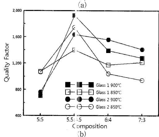
그림 3. 코디어라이트/글라스(5/5) 조성의 소결 온도 변화에 따른 유전율 및 품질계수.
