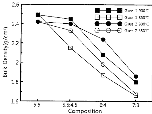
그림 2. 코디어라이트/글라스(5/5) 조성의 소결 온도 변화에 따른 밀도.
