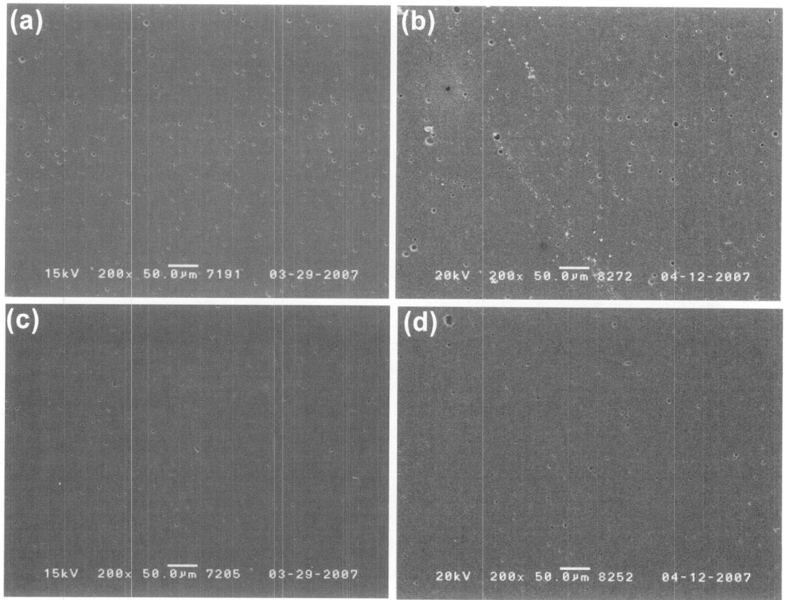
그림 5. 코디에라이트/글라스 1(5/5) 시편의 소성온도 및 유지시간 변화에 따른 시편의 미세구조: (a) 900°C 2시간 (b) 875°C 2시간 (c) 850°C 2시간 (d) 875°C 5분.
