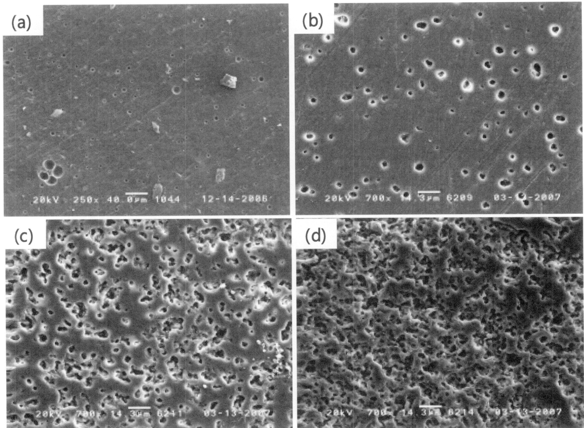
그림 4. 900°C 2시간 소결한 코디에라이트/글라스 1 조성 변화에 따른 시편의 미세구조: (a) 5:5 (b) 5.5:4.5 (c) 6:4 (d) 6.5:3.5.
