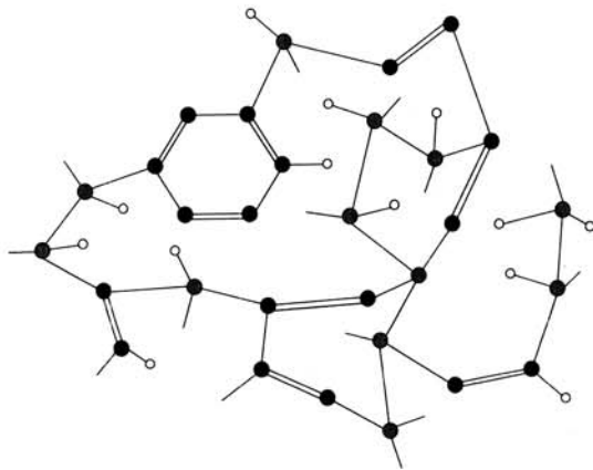
그림 2. Hydrogenated DLC (a-C:H) 박막의 결합 구조, ● sp^3 결합 탄소 원자, ● sp^2 결합 탄소 원자, ○ 수소 원자. Fig. 2. Bonding structure of hydrogenated DLC (a-C:H) thin film, ● carbon atoms of sp^3 bonding, ● carbon atoms of sp^2 bonding, ○ hydrogen atoms.
