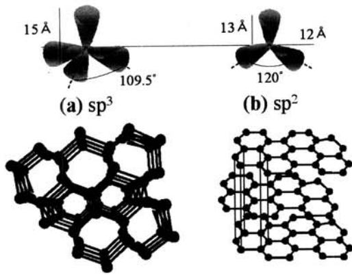
그림 1. Sp hybridization 결합과 결정구조, (a) sp^3 다이아몬드, (b) sp^2 흑연. Fig. 1. Sp hybridization bonding and crystal structure, (a) sp^3 diamond, (b) sp^2 graphite.
