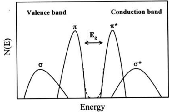
그림 3. DLC 박막의 에너지밴드 다이어그램[6]. Fig. 3. Energy band diagram of DLC thin film.
