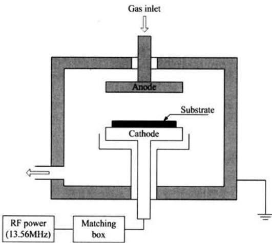
그림 4. 실험에 사용된 capacitive-coupled cathode 타입 RF PECVD 시스템의 개략도.
