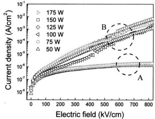
그림 5. RF 파워에 따른 DLC 박막의 전류-전압 특성.
