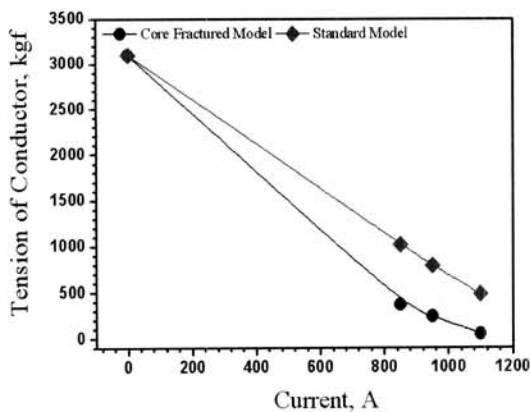
그림 8. 전류에 대한 전선의 장력 변화 거동. Fig. 8. Change of tension with current.
