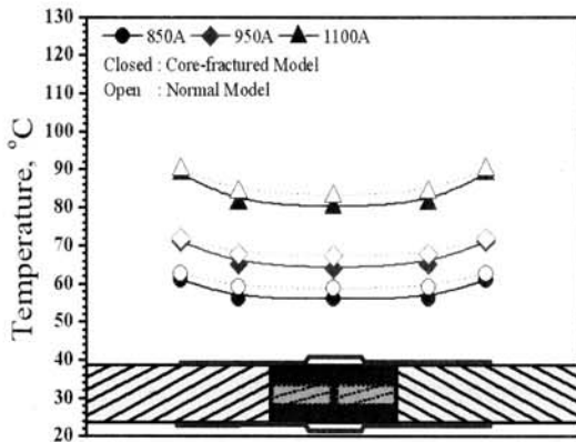
그림 5. Al 슬리브의 온도분포. Fig. 5. Distribution of Al sleeve temperature.
