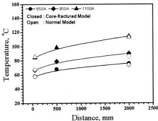
그림 4. 도체의 온도 분포.
