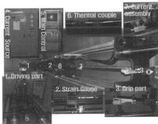
그림 1b). 가공전선의 탄성계수와 선팽창계수 측정.
