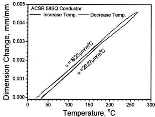
그림 5. ACSR 58 mm 2 가공송전선의 온도-신율 곡선.
