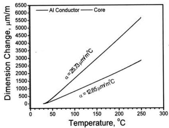
그림 4. 알루미늄도체의 온도-신율 곡선.
