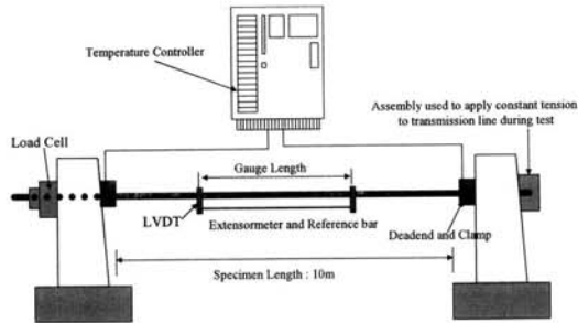
그림 1a). 가공송전선의 탄성계수와 선팽창계수를 측정하기 위한 개략도.
