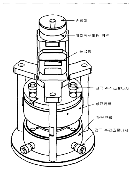
그림 3. 검증을 위하여 제작된 유전율 측정용 3-전극 시스템.
