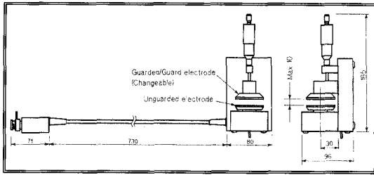
그림 1. 상품화된 유전율 측정용 cell의 구조. Fig. 1. Structure of commercialized dielectric test cell assemble.
