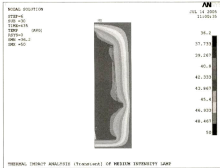
그림 21. 온도분포도(시간 = 435분). Fig. 21. Temperature result(time = 435 min).
