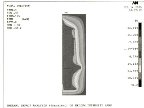
그림 18. 온도분포도(시간 = 195분).
