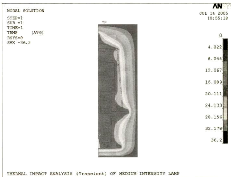
그림 16. 온도분포도(시간 = 0분).
