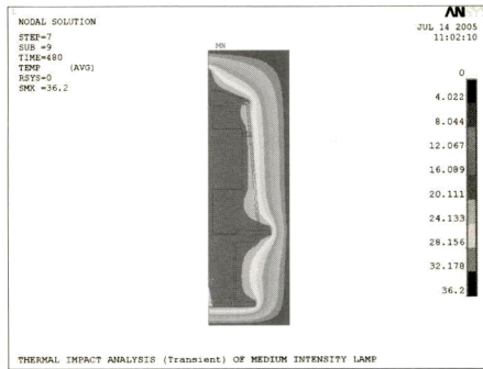
그림 22. 온도분포도(시간 = 485분) Fig. 22. Temperature result(time = 485 min).
