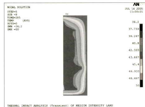
그림 20. 온도분포도(시간 = 285분).
