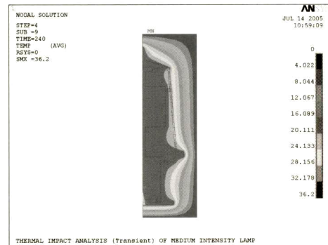
그림 19. 온도분포도(시간 = 240분).
