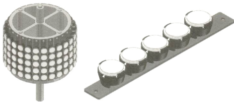
그림 2. 3차원 LED 모듈 모델링. (고휘도 LED 5단) Fig. 2. 3-dimensional LED module modeling. (5-layer power LED)
