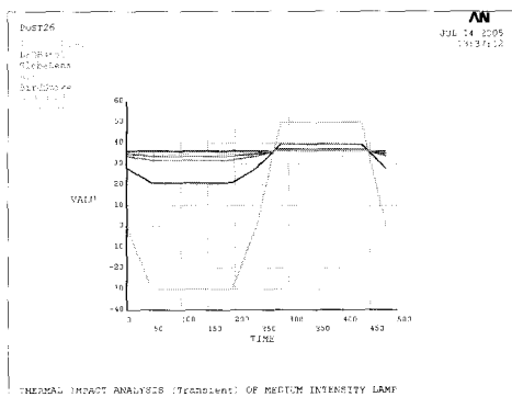
그림 23. 과도(Transient) 온도반응특성. Fig. 23. Transient temperature response.
