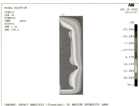
그림 17. 온도분포도(시간 = 45분).
