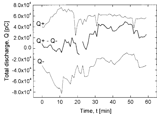
그림 11. 구리의 총 방전 전하량 Q. Fig. 11. Total discharge Q of copper.
