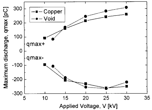
그림 5. 최대 방전 전하량 q_{max} 의 전압의존성. Fig. 5. Voltage dependence of q_{max} .
