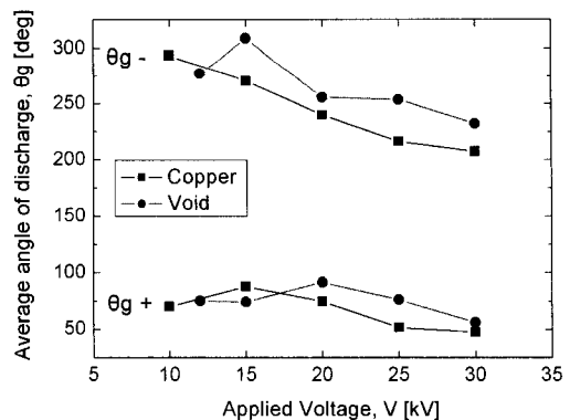
그림 7. 평균 방전 발생 위상각 \theta_g 의 전압의존성. Fig. 7. Voltage dependence of \theta_g .
