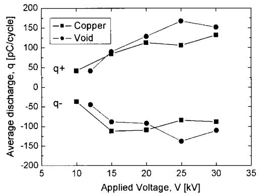
그림 6. 평균 전하량 q의 전압의존성. Fig. 6. Voltage dependence of q.
