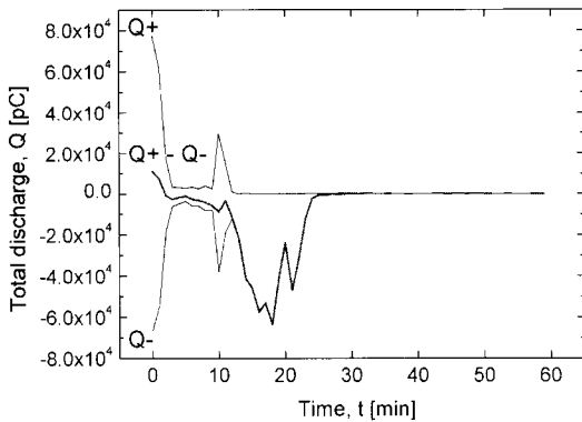
그림 10. 보이드의 총방전 전하량 Q. Fig. 10. Total discharge Q of void.
