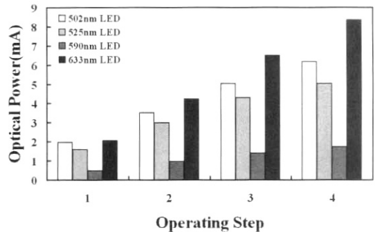
그림 7. LED의 스텝에 따른 광출력의 변화.
