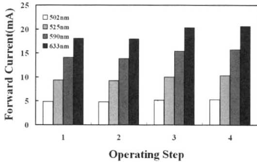
그림 5. 스텝에 따른 전류 변화.
