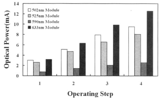
그림 6. 광모듈의 스텝에 따른 광출력의 변화.
