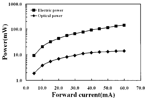
그림 3. 기기의 출력 특성. Fig. 3. Characteristics of power of equipment.
