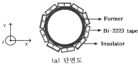
(a) 단면도
