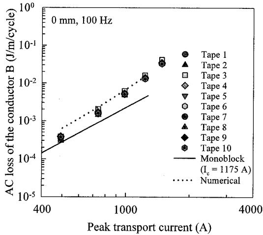
그림 7. 도체 B에서 교류손실의 접촉위치 의존성. Fig. 7. AC loss vs. peak transport current for different contact positions in the conductor B.
