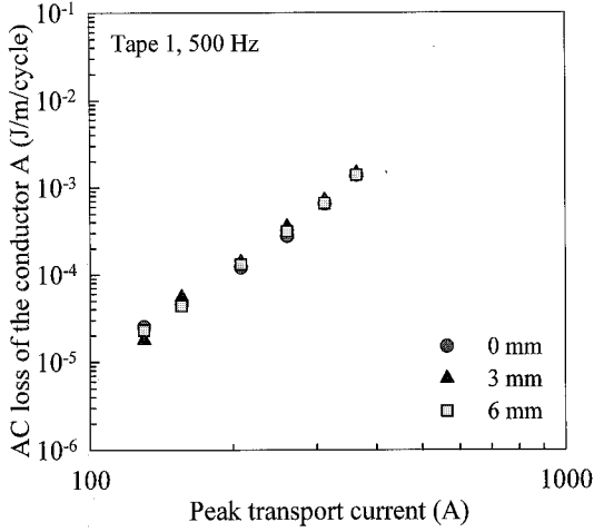
그림 4. 도체 A에서 교류손실의 전압리드 배열 의존성.
