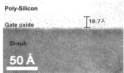
그림 2. 0.11 \mu\text{m} CMOS 기술로 제작된 소자의 HR-TEM 사진.
