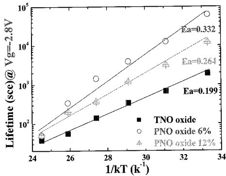
그림 9. 스트레스 온도에 따른 NBTI 수명시간의 Arrhenius plot.
