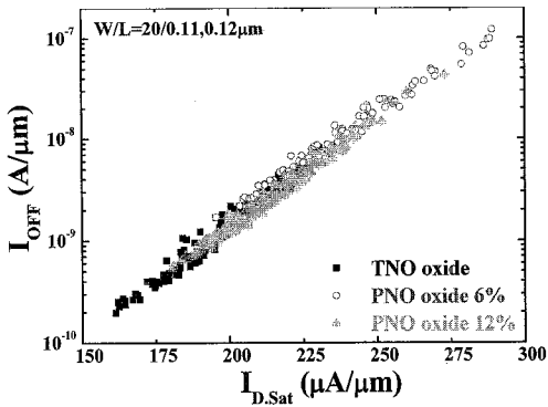
그림 3. 게이트 산화막 성장 방법에 따른 I_{D,Sat} vs. I_{OFF} 특성.
