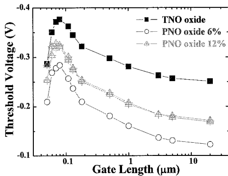
그림 4. 게이트 산화막 성장 방법에 따른 V_{th} roll-off 특성.
