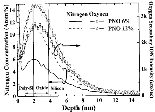
그림 10. Plasma nitride oxide에서 nitrogen과 oxygen의 SIMS profile.
