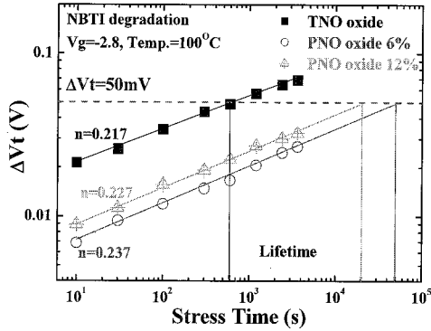
그림 7. 게이트 산화막 성장 방법에 따른 PMOSFET의 Bias Temperature Instability 열화 특성. Fig. 7. Comparison of Bias temperature instability degradation of PMOSFET between gate oxidation methods.
