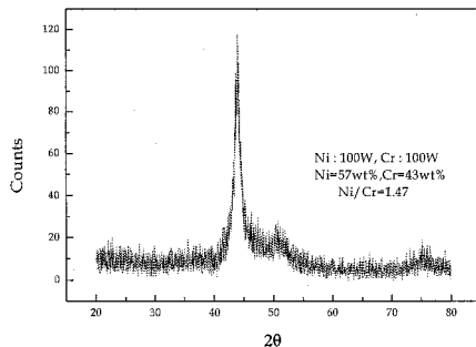
그림 5. Ni/Cr 성분함량 변화에 따른 XRD. Fig. 5. XRD with Ni/Cr compositions.
