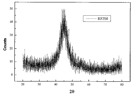
그림 9. DC/RF Power변화에 따른 XRD. Fig. 9. XRD with DC/RF power.
