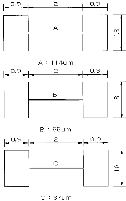
그림 1. 박막저항의 단위Cell 설계도.
