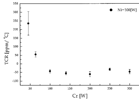
(a) Cr추 증가 power에 따른 TCR(Ni=100 W)
