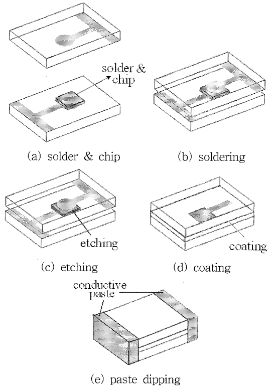
그림 1. 제조 과정.
