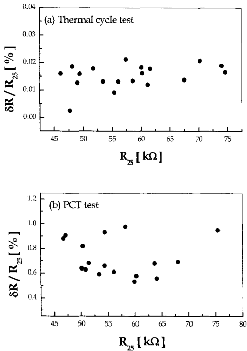
그림 3. 신뢰성 시험후 저항 변화. Fig. 3. Resistance variation after thermal cycling/PCT test.
