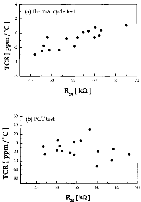
그림 4. 신뢰성 시험후 저항온도계수 특성. Fig. 4. TCR after thermal cycling or PCT test.
