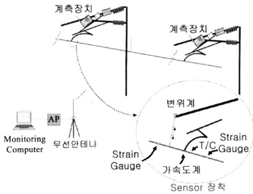
그림 2. 현장시험을 위한 전차선로 실시간 계측시스템의 설치방법. Fig. 2. Installation method of real-time data acquisition system for a field test.
