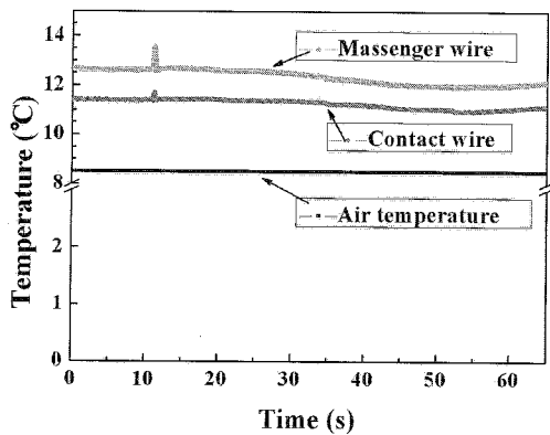
그림 5. 전차선과 조가선의 온도특성.
