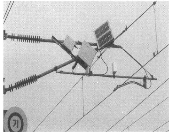
그림 3. 실시간 계측시스템의 사진. Fig. 3. Picture of the real-time data acquisition system.
