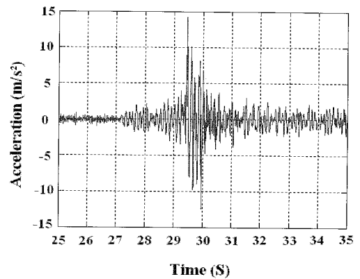
그림 7. 가속도 측정 결과.
