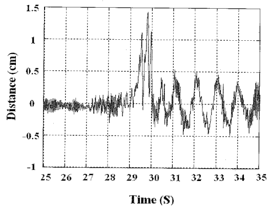
그림 6. 변위 측정 결과.
