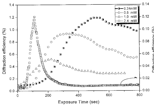
그림 6. Ag/As_{40}Ge_{10}Se_{15}S_{35} 박막에서의 회절효율.
