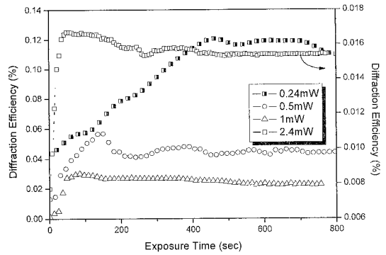
그림 7. As_{40}Ge_{10}Se_{15}S_{35}/Ag/As_{40}Ge_{10}Se_{15}S_{35} 박막에서의 회절효율.
