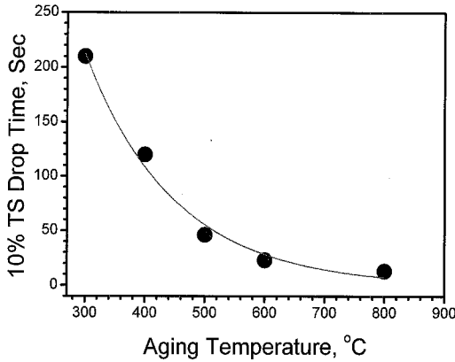
그림 5. 열화온도에서 인장강도의 10%저하에 소요되는 시간.
