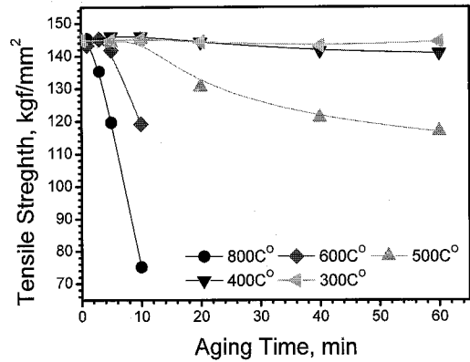
그림 4. 열화에 의한 아연도금강선의 인장강도 변화. Fig. 4. Tensile strength of core by aging.
