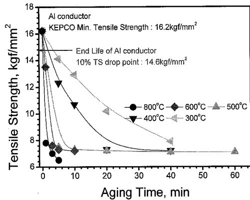
그림 3. 열화에 의한 알루미늄도체 인장강도 변화. Fig. 3. Tensile strength of Al conductor by aging.
