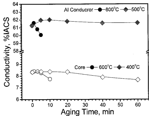
그림 8. 열화에 의한 알루미늄도체와 아연도금강선의 전기전도도 변화.
