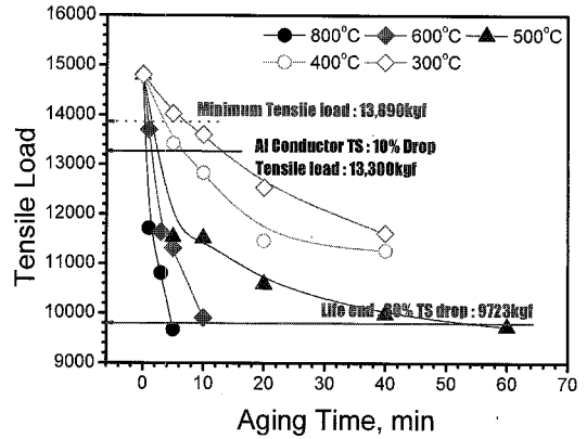
그림 6. 열화에 의한 ACSR 410 mm 2 가공전선 인장하중.
