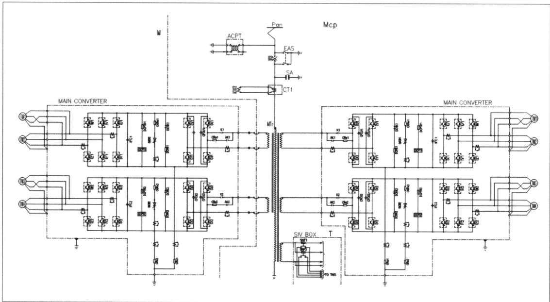
그림 1. 주회로시스템.
