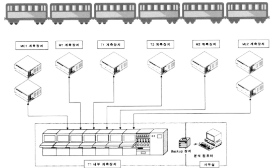
그림 5. 탈팅차량 전체 시스템 구성도. Fig. 5. Overall system composition of TTX.
