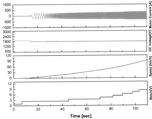
그림 11. 점진적 역행시험 파형. Fig. 11. Wave of gradually powering test.
