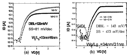
그림 3. SONOS 메모리의 전달 특성 (a) 게이트 길이와 폭이 W/L=33 nm/46 nm인 LDD 공정을 수행한 소자 (b) 게이트 길이와 폭이 W/L=34 nm/31 nm인 LDD 공정을 수행하지 않은 소자
