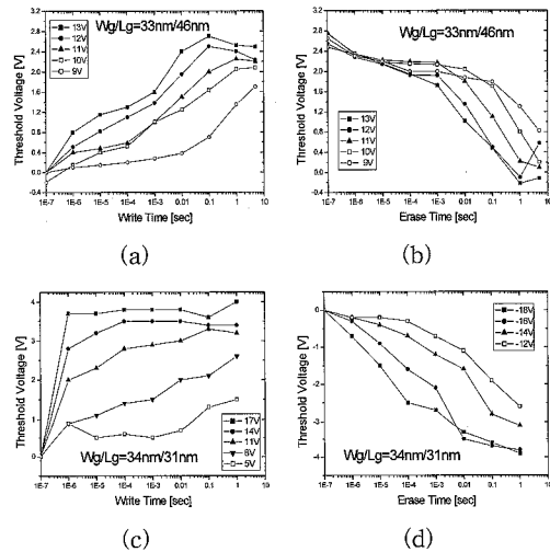
그림 4. SONOS 메모리 소자의 전압에 따른 쓰기 (a)(c)와 소거(b)(d) 특성: (a)(b) LDD 공정을 수행한 채널 W/L가 33/ 46 nm 이고 ONO 두께가 2 /7 /9 nm인 소자, (c)(b) LDD 공정 없고 W/L= 33/ 31 nm 이고 ONO = 4.5 /9.3 /6.5 nm인 소자.
