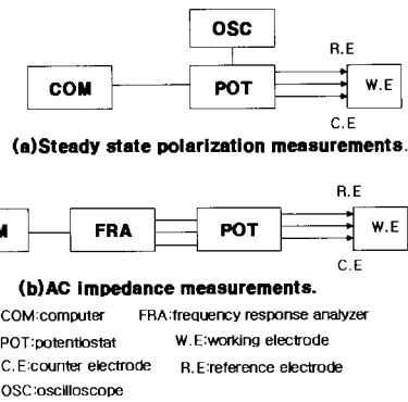
그림 1. 정상 분극과 임피던스 측정의 블록다이어그램.
