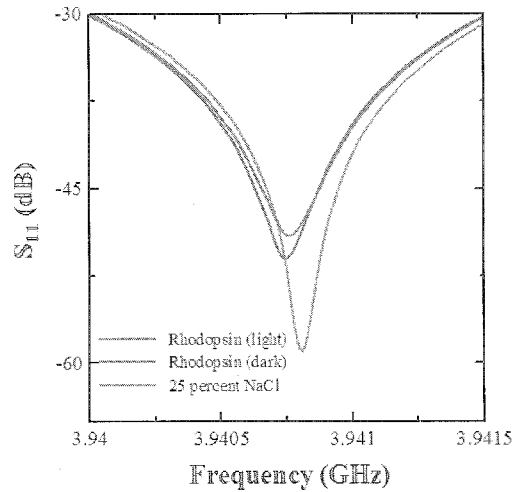
그림 4. 밝은 환경과 어두운 환경에서 NpSR II의 마이크로파 반사계수 ( S_{11} ). Fig. 4. Microwave reflection-coefficient ( S_{11} ) of NpSR II in light and dark.
