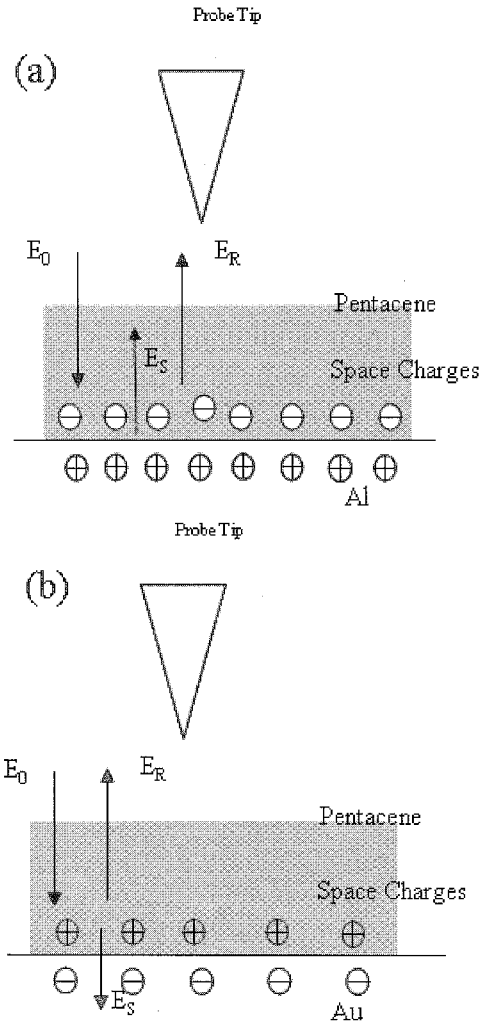
그림 2. Al과 Au 기저 금속으로부터 잉여 전하의 이동을 나타낸 (a) pentacene/Al 과 (b) pentacene/Au 소자의 개략도.
