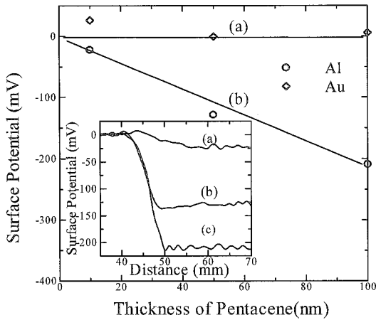
그림 5. Kelvin-probe 방법으로 측정한 (a) pentacene/Au 와 (b) pentacene/Al 소자의 pentacene 두께에 따른 surface potential 변화. 삽입한 그림은 pentacene/Al 소자의 실제 surface potential 값이다. (a) 10 nm, (b) 50 nm, (c) 100 nm.
