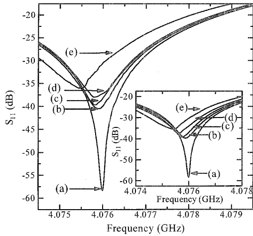
그림 3. pentacene/Al 과 pentacene/Au(삽입한 그림) 소자의 마이크로웨이브 반사계수 S_{11} : (a) glass (b) Al(or Au) 전극 (c) 10 nm pentacene (d) 50 nm (e) 100 nm.
