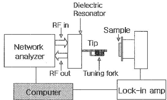
그림 1. 거리 조절 시스템을 가진 마이크로파 근접장 현미경의 개략도.
