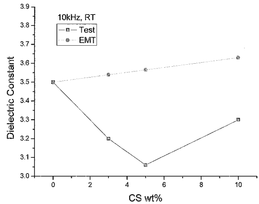
그림 5. CS 조성에 따른 유전율 특성곡선.
