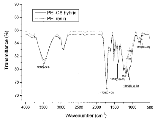
그림 2. PEI 수지와 PEI-CS졸(10 wt%) 하이브리드 시편의 FT-IR 분석.
