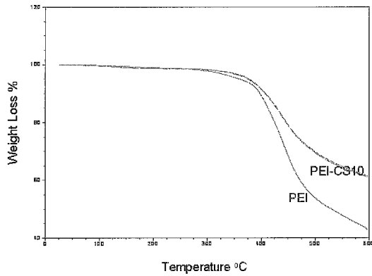
그림 3. PEI 수지와 PEI-CS졸(10 wt%) 하이브리드 시편의 TGA 분석
