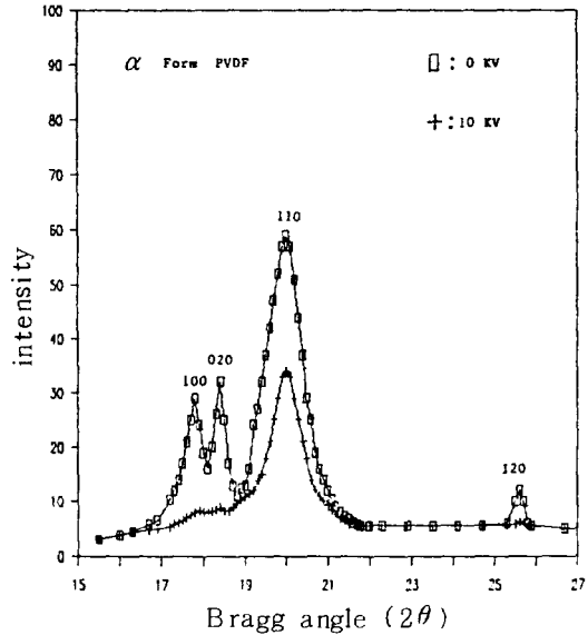
그림 4. 코로나 전압 변화에 따른 \alpha 형 시료의 X-선 회절도
