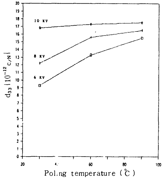
그림 7. \alpha + \beta 형 PVDF에 대한 압전계수의 분극온도 의존성
