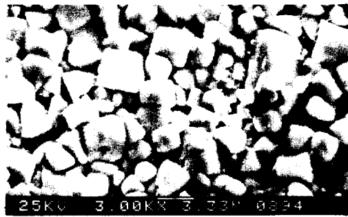
그림 3. 소결된 PZT501A 세라믹스의 미세구조 Fig 3. Microstructure of sintered PZT 501A ceramics
