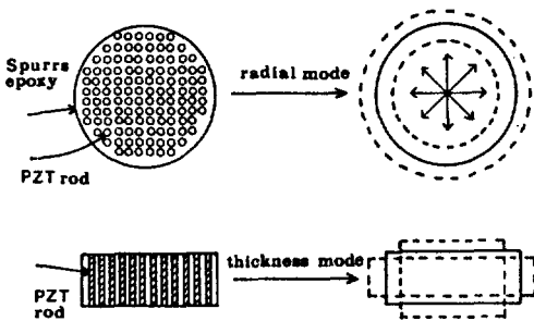
그림 10. 경방향 및 두께방향의 공진모드 Fig 10. Resonance mode of radial and thickness direction
