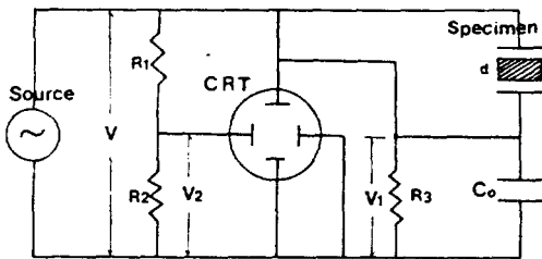
그림 5. Sawyer-Tower 회로도 Fig 5. Sawyer-Tower circuit for D-E measurement
