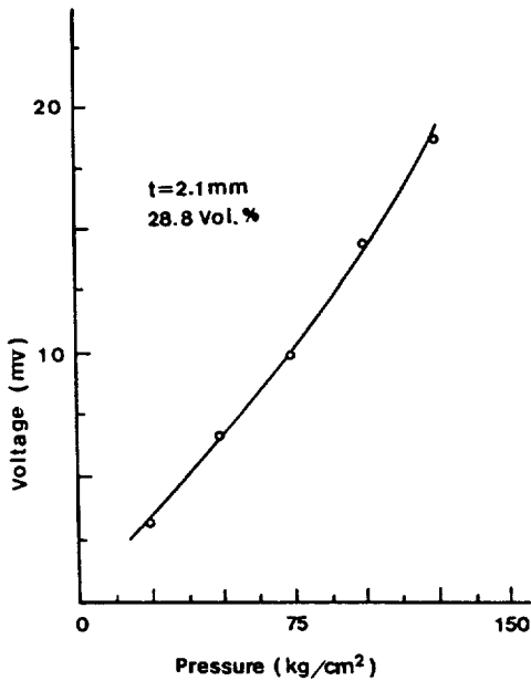
그림 16. 압력변화에 따른 유증발생전압 Fig 16. Generated voltage under oil pressure to the oil press
