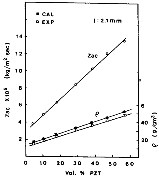
그림 8. PZT체적비에 따른 음향임피던스와 밀도
