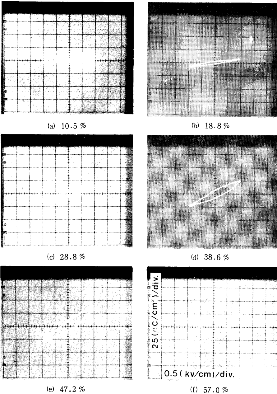
그림 9. PZT 체적비 변화에 따른 D-E곡선 Fig 9. D-E curve to the PZT volume percent
