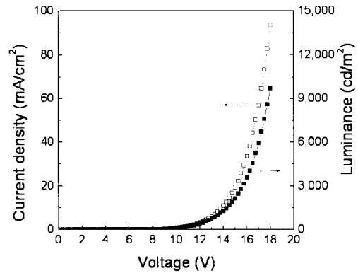
그림 3. Ba(10 nm)/Ag(8 nm)를 투명 음극으로 사용한 전면발광 OLED의 전압에 따른 전류밀도 및 휘도 변화.
