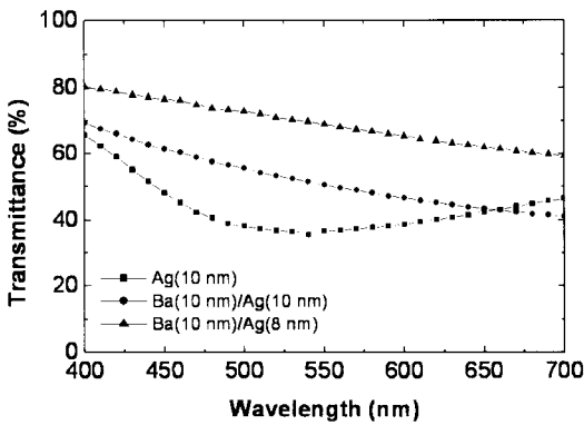
그림 2. Ba/Ag 및 Ag 층의 투과도 변화. Fig. 2. Transmittance variation of the Ba/Ag and Ag layered cathodes.
