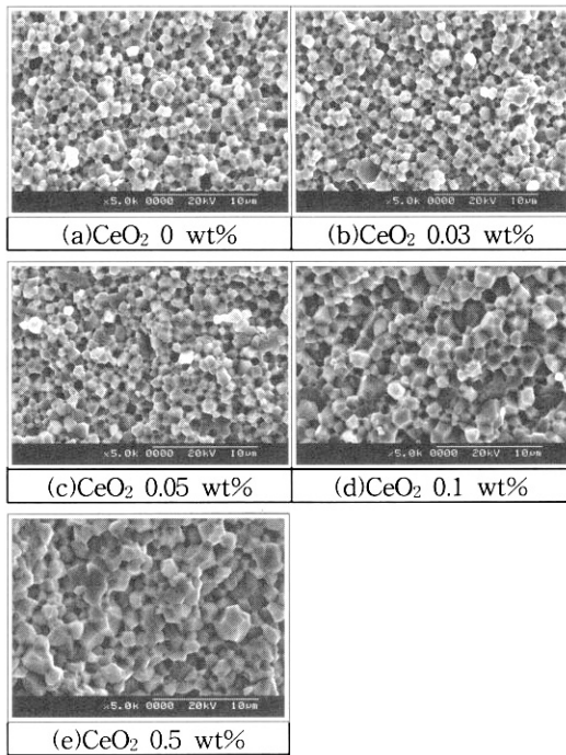
그림 3. 1310 °C에서 2시간 소결한 PSN-PMN-PZT의 SEM파단면: (a) CeO 2 =0 wt%, (b) 0.03 wt%, (c) 0.05 wt%, (d) 0.1 wt%, (e) 0.5 wt%.
