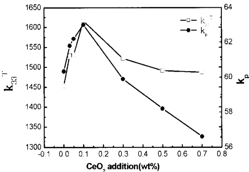
그림 4. CeO 2 첨가량에 따른 전기기계결합계수 k_p 와 유전 상수 K_{33}^T .
