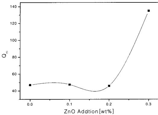
그림 6. ZnO첨가에 따른 기계적 품질계수(Q m ). Fig. 6. Mechanical quality factor (Q m ) varied with ZnO amount.
