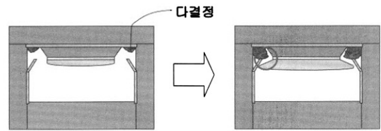
그림 7. 다결정 실리콘 카바이드의 성장 양상. Fig. 7. The formation of polycrystalline region in SiC growth process.
