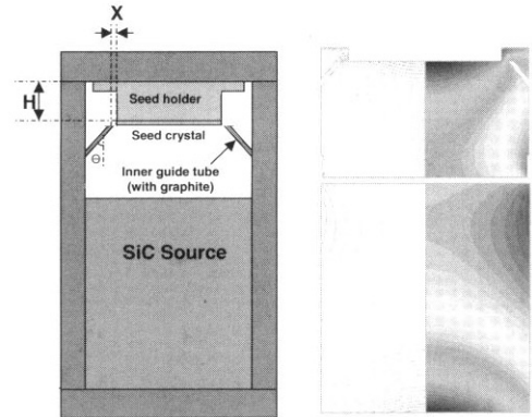
그림 2. 실리콘 카바이드 성장에 사용하는 전형적인 도가니 구조와 시뮬레이션을 통하여 얻은 온도분포.
