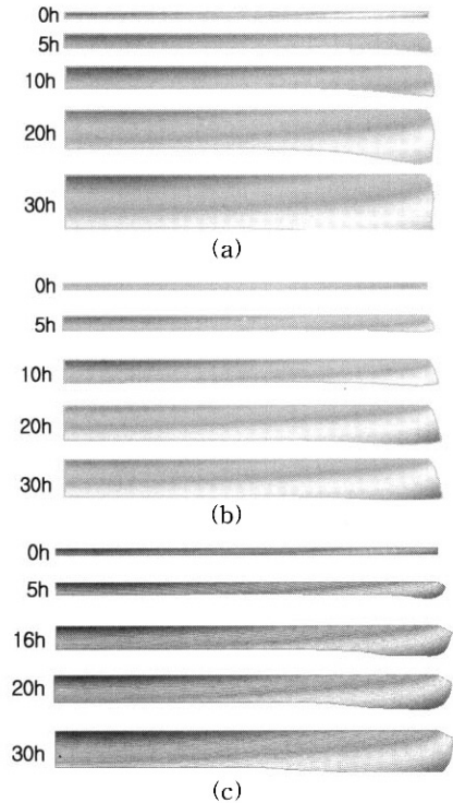
그림 3. 다양한 각도로 구성되어 있는 trapezoid 형상의 seed holder에 대한 시뮬레이션 결과.
