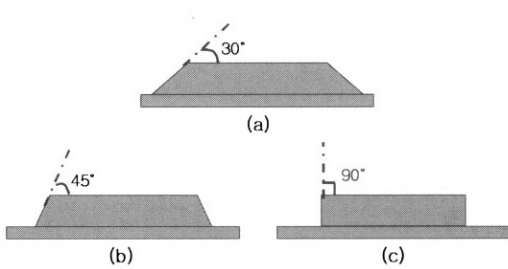
그림 1. 다양한 각도로 구성되어 있는 trapezoid 형상의 seed holder.
