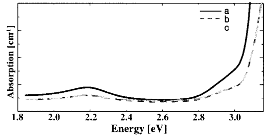
그림 9. Seed holder의 각도에 따라 성장된 실리콘 카바이드 단결정의 UV-Visible Spectroscopy 특성.
