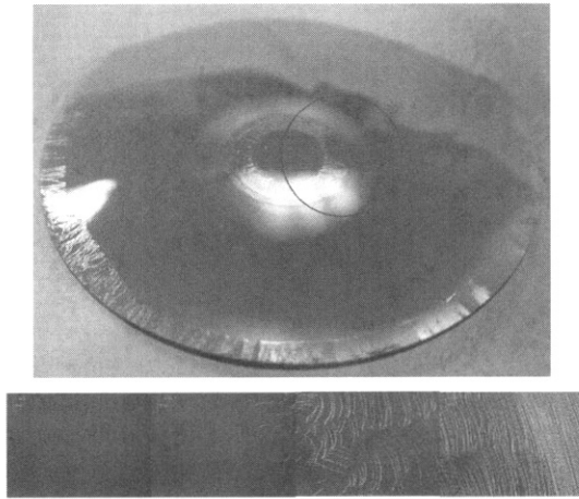
그림 11. 단결정 잉곳의 성장점의 현미경 사진. Fig. 11. Microscope images of the growth point of single crystal ingot.
