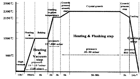
그림 5. 실리콘 카바이드 단결정의 공정 조건. Fig. 5. The process condition for SiC single crystal growth.
