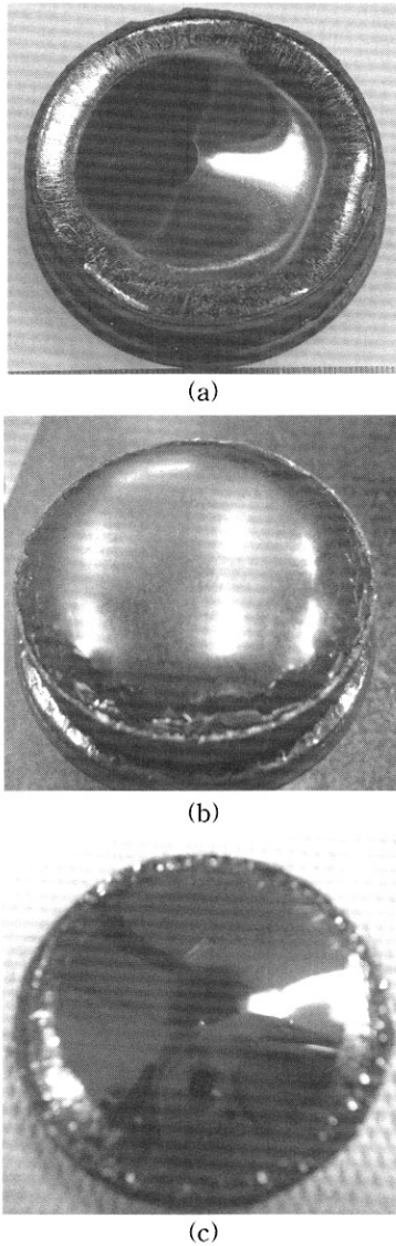
그림 6. Seed holder의 각도에 따라 PVT법으로 성장된 실리콘 카바이드 단결정 ingot. (a) = 30°, (b) = 45°, (c) = 90° Fig. 6. Silicon carbide single crystal ingot grown by PVT method with different angles of seed holder. (a) = 30°, (b) = 45°, (c) = 90°
