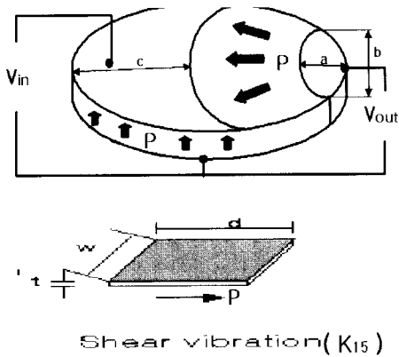
그림 2. Crescent형 압전변압기의 구조 및 전단변위 진동모드. Fig. 2. Structure of Crescent input type piezoelectric transformer & Shear vibration mode.
