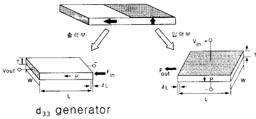
그림 1. Rosen형 압전변압기의 원리. Fig. 1. Principle of Rosen type piezoelectric transformer.
