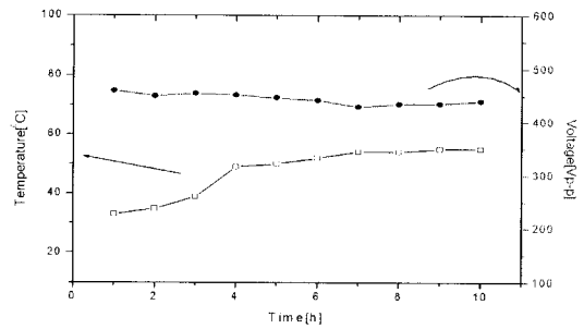
그림 13. CCFL의 전압 및 온도특성. Fig. 13. Characteristic of voltage and temperature for CCFL.
