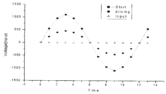
그림 12. CCFL의 초기전압 및 운전전압. Fig. 12. Starting voltage and driving voltage of CCFL
