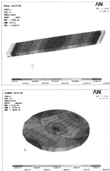
그림 3. Rosen형과 Crescent형 압전변압기의 유한 요소 해석.
