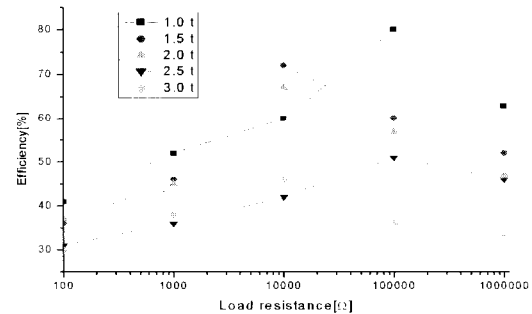
그림 9. 부하저항 변화에 따른 효율(두께). Fig. 9. Efficiency by changes of load resistance (thickness).
