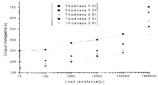
그림 7. 부하저항 변화에 따른 출력전압. Fig. 7. Output voltage by changes of load resistance.
