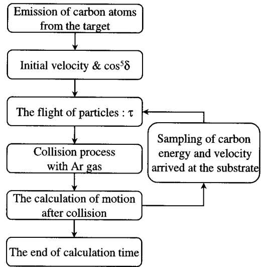
그림 3. 레이저 용삭법에 의한 플라즈마 시뮬레이션 순서도.
