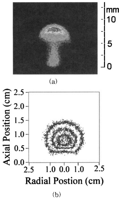
그림 4. 질소 기체 P=10 Pa 압력하에서 530 ns 경과시의 레이저에 의해 발생된 플라즈마 형상. (a) C_2 와 CN 입자의 발광 CCD 화상, (b) 탄소원자의 시뮬레이션 결과.
