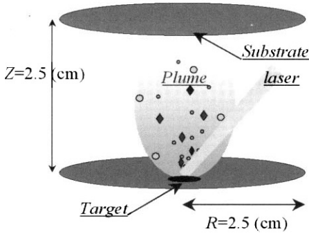
그림 1. 방전 챔버 모델. 방전 챔버의 높이 Z=2.5 cm, 챔버의 반경 R=2.5 cm, 가스압력 P=\text{Vacuum} ( 10^{-5} Pa)~66 Pa. Fig. 1. The model of discharge chamber. The height of chamber Z=2.5 cm, the radius R=2.5 cm, and the pressure P=\text{Vacuum} ( 10^{-5} Pa) ~66 Pa.
