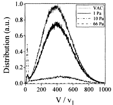
그림 7. 기판에 퇴적된 탄소 원자의 속도 분포. Fig. 7. The velocity distribution of carbon particles deposited upon the substrate. V is velocity and v_1 is the velocity of carbon particle with 0.01 eV energy.
