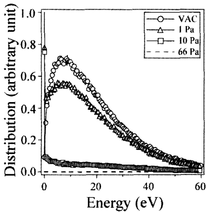
그림 6. 기판에 도달한 탄소 원자의 에너지 분포. Fig. 6. Carbon energy distributions deposited upon the substrate.
