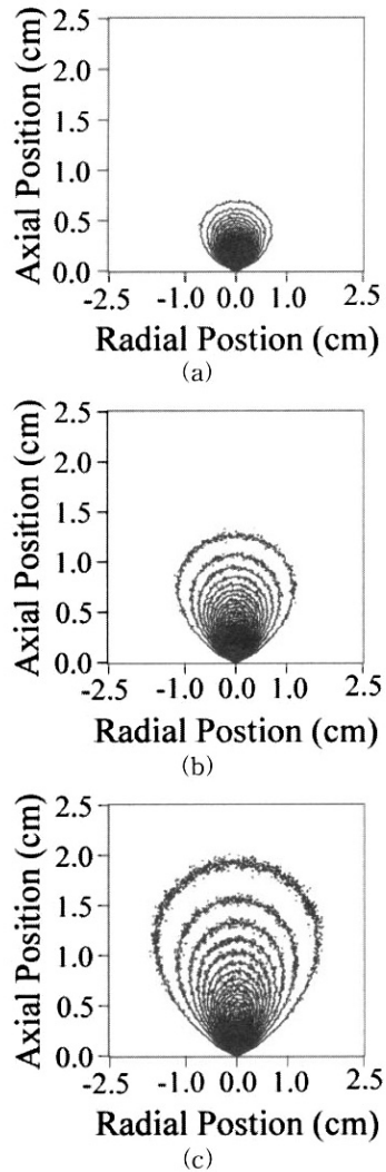
그림 5. Ar 기체압력 P=1 Pa 조건하에서의 탄소 입자의 진전 과정. (a) 100 ns, (b) 500 ns, (c) 100 \mu s. 각각의 등고선은 최대값(6,250)과 최소값(125)을 50등분한 것.
