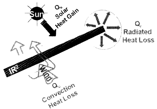
그림 3. 가공송전선과 열적환경.
