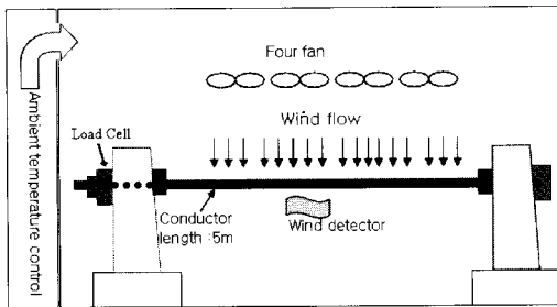
그림 1. 환경챔버 개략도.
