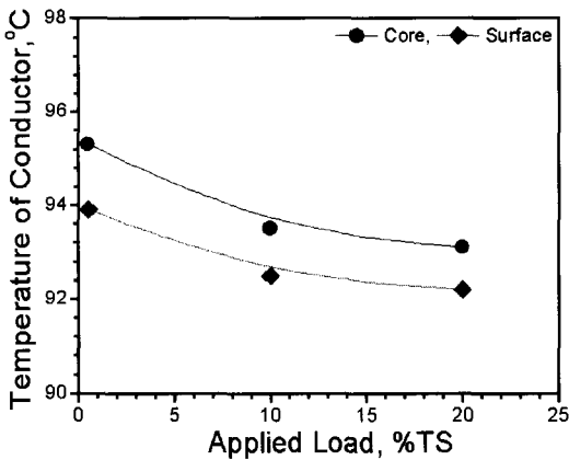
그림 5. 850 A, 무풍 상태에서 장력에 따른 전선 온도.
