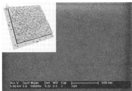
그림 7. 1.5 sccm 산소 유량비 하에서 성막된 IZO 박막의 SEM 과 AFM 표면 사진.
