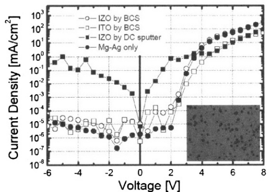
그림 8. 박스 캐소드 스퍼터 및 DC 스퍼터를 이용해 성막한 상부 캐소드 전극을 가진 전면 발광 OLED의 전류-전압 특성 및 EL 이미지.
