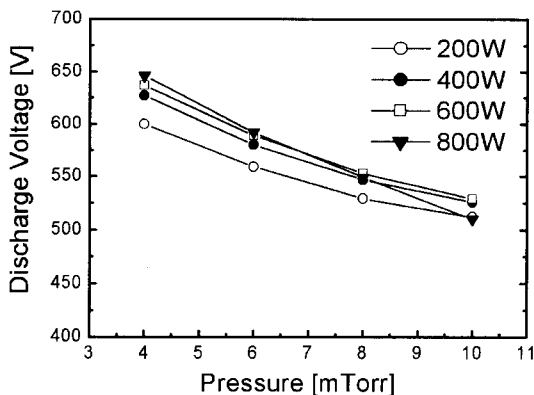
그림 2. 박스 캐소드 전 내의 작업 압력의 증가에 따른 방전 전압 변화.
