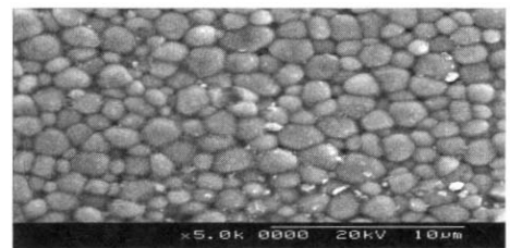
(d) 5 mol%
