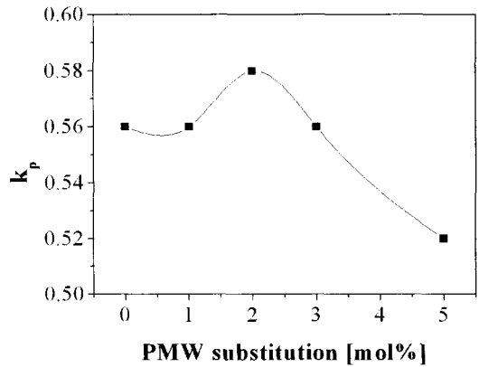
그림 4. PMW치환에 따른 전기기계결합계수(k p ). Fig. 4. Electromechanical coupling factor(k p ) with PMW substitution.
