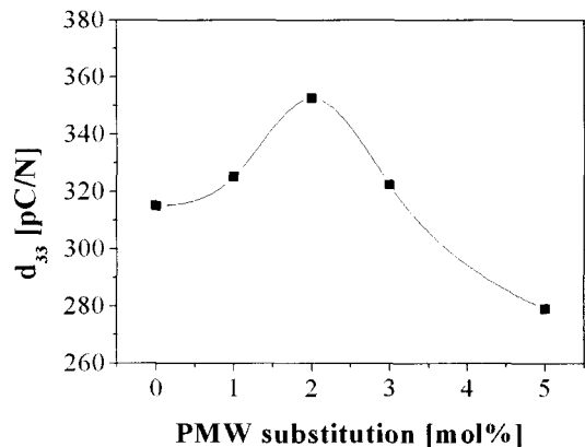
그림 5. PMW치환에 따른 압전상수(d 33 ). Fig. 5. Piezoelectric constant(d 33 ) with PMW substitution.
