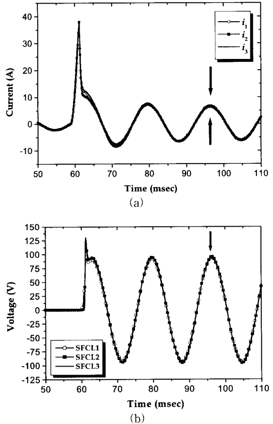
그림 5. 하나의 강자성체 철심을 사용한 SFCL의 전기적 특성(전원 전압 : 220 V rms ). Fig. 5. Quench properties of SFCL units using a single ferromagnetic core(applied voltage: 220 V rms ). (a) Current curves of three SFCLs. (b) Voltage curves of three SFCLs.
