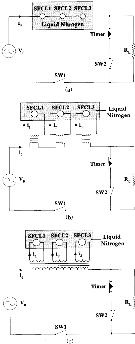
그림 1. 실험 회로 구성도.
