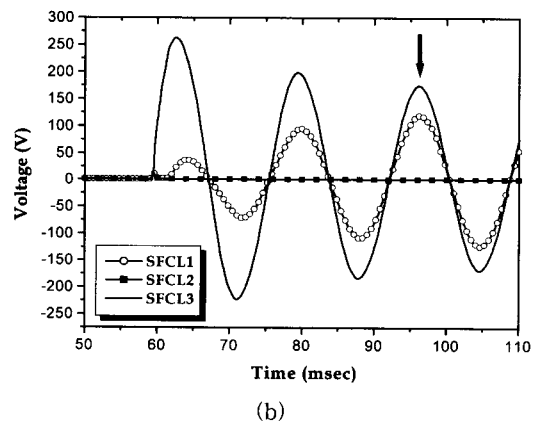
그림 3. 단순 직렬 연결된 SFCL의 전기적 특성 (전원 전압 : 220 V rms ).
