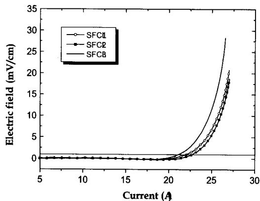
그림 2. 초전도 소자의 I-V 곡선. Fig. 2. I-V curves of individual SFCL units.
